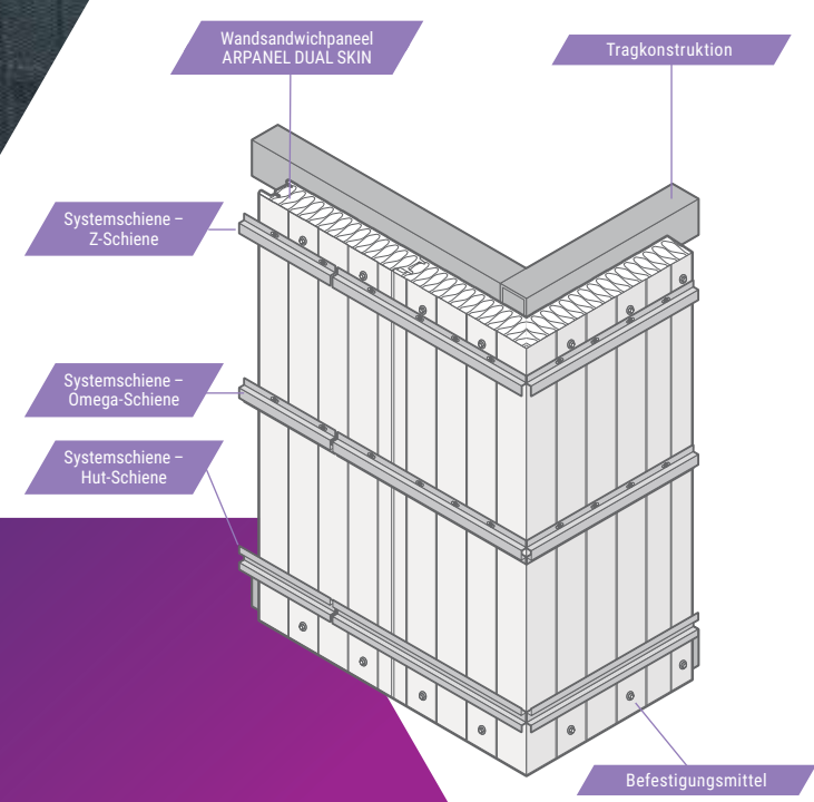
Wandaufbau aus Sandwichpaneelen für das ARPANEL DUAL SKIN System – vertikale Montage
